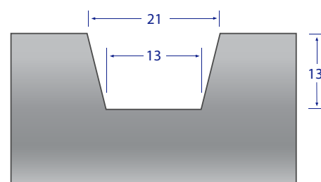
Canal para mesa de deslizamento
