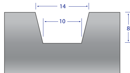
Canal para mesa de deslizamento
