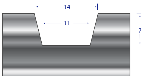
Canal para polias
