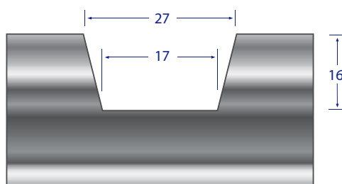
Canal para polias
